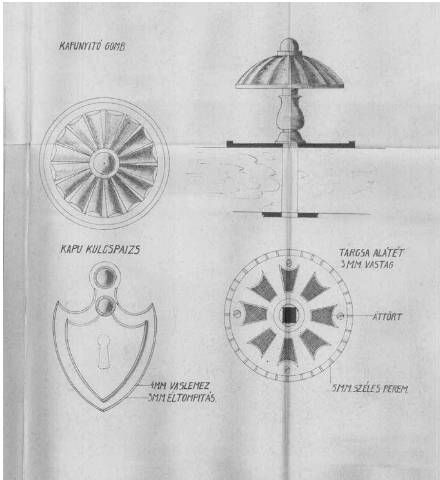
A bejárati ajtó és a szélfogó vasalatainak tervrajzai, 1951
