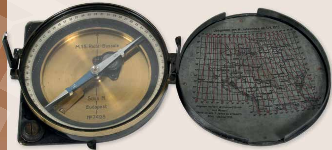
1915 M ütegszögmérő. A Budapesten gyártott eszköz fedelének belsején a mágneses elhajlást mutató ábra található
